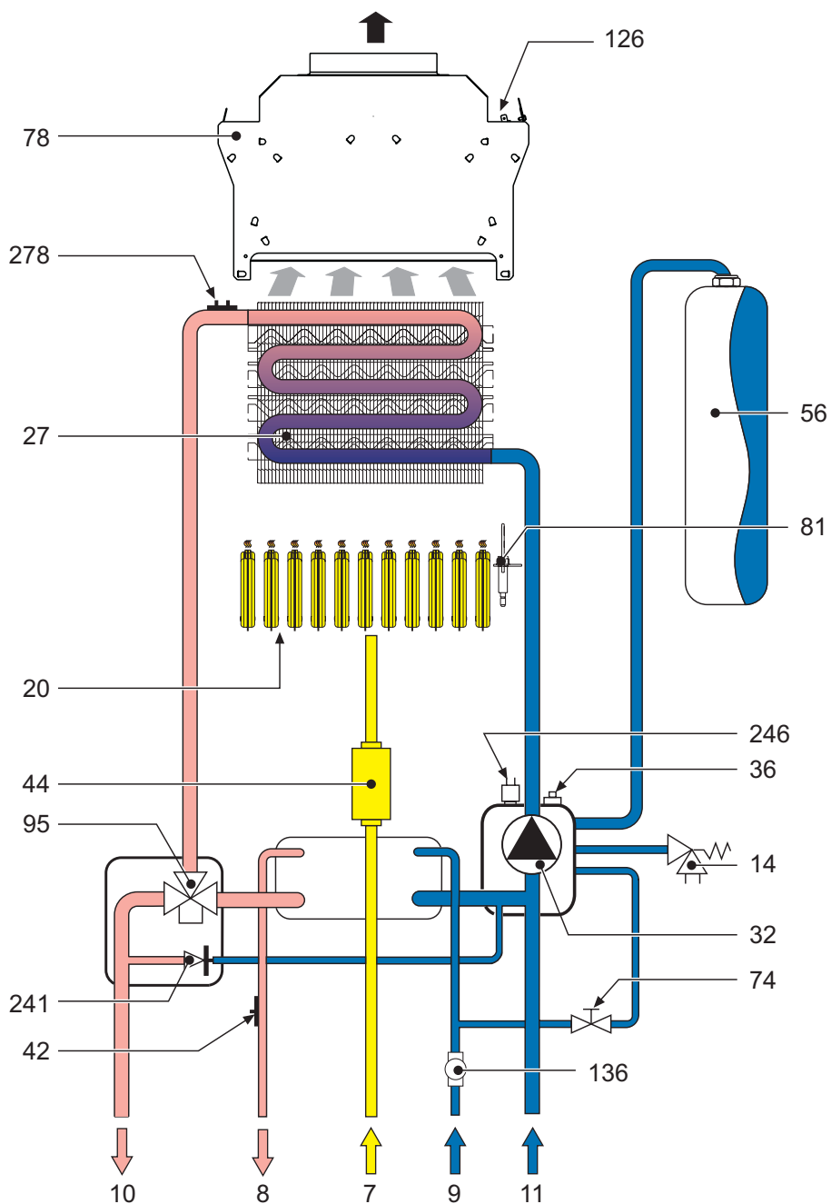
fig. 27 - Circuito idraulico
