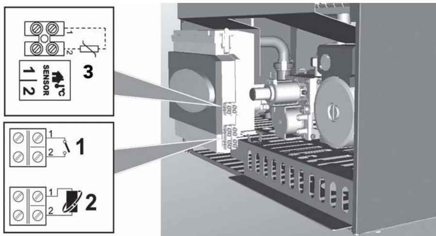
fig. 21 - Accesso alla morsettiera
