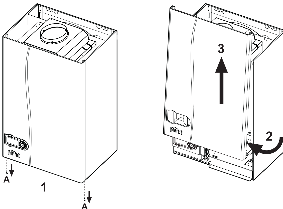
fig. 24 - Apertura mantello
