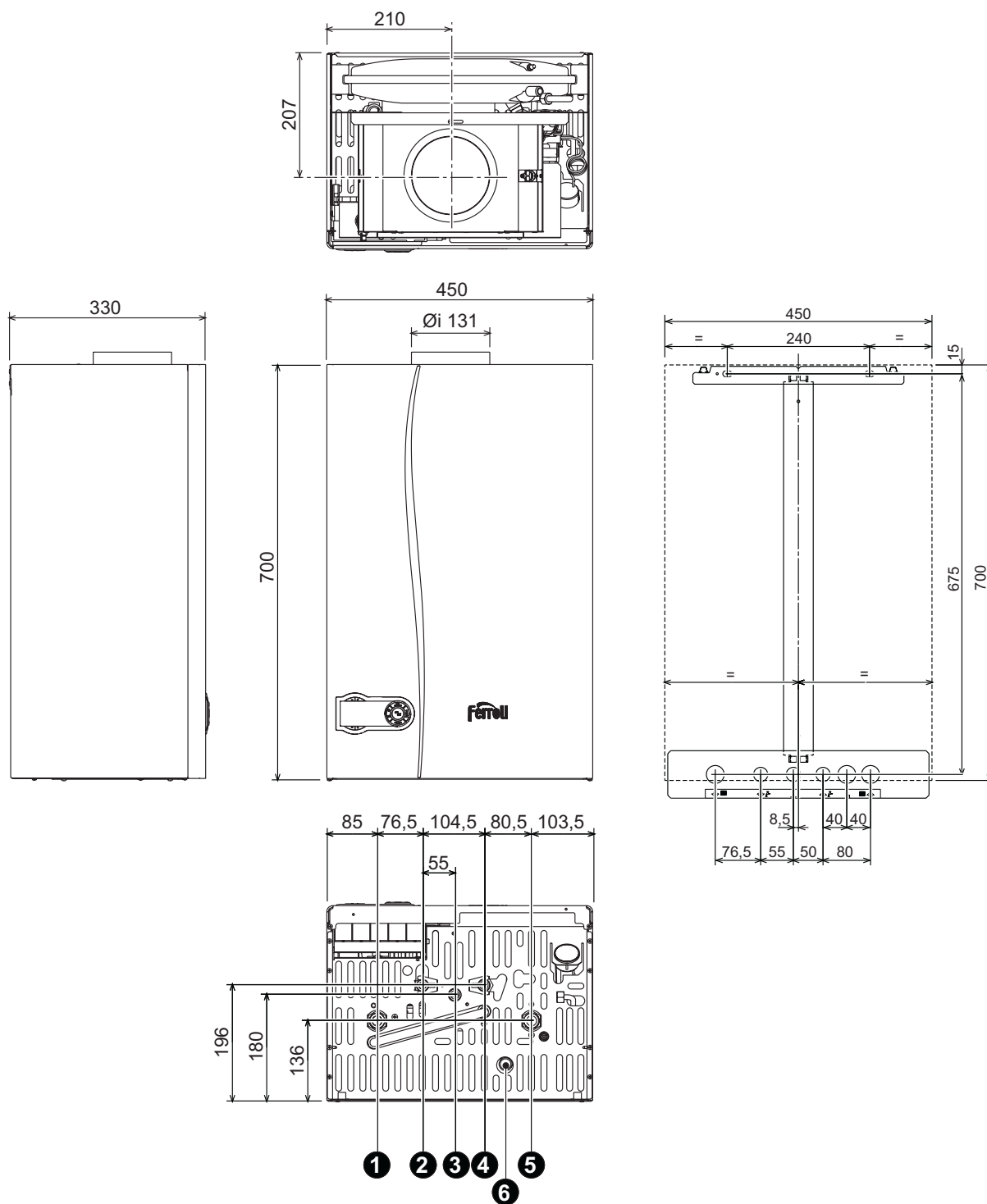
fig. 25 - Dimensioni e attacchi
