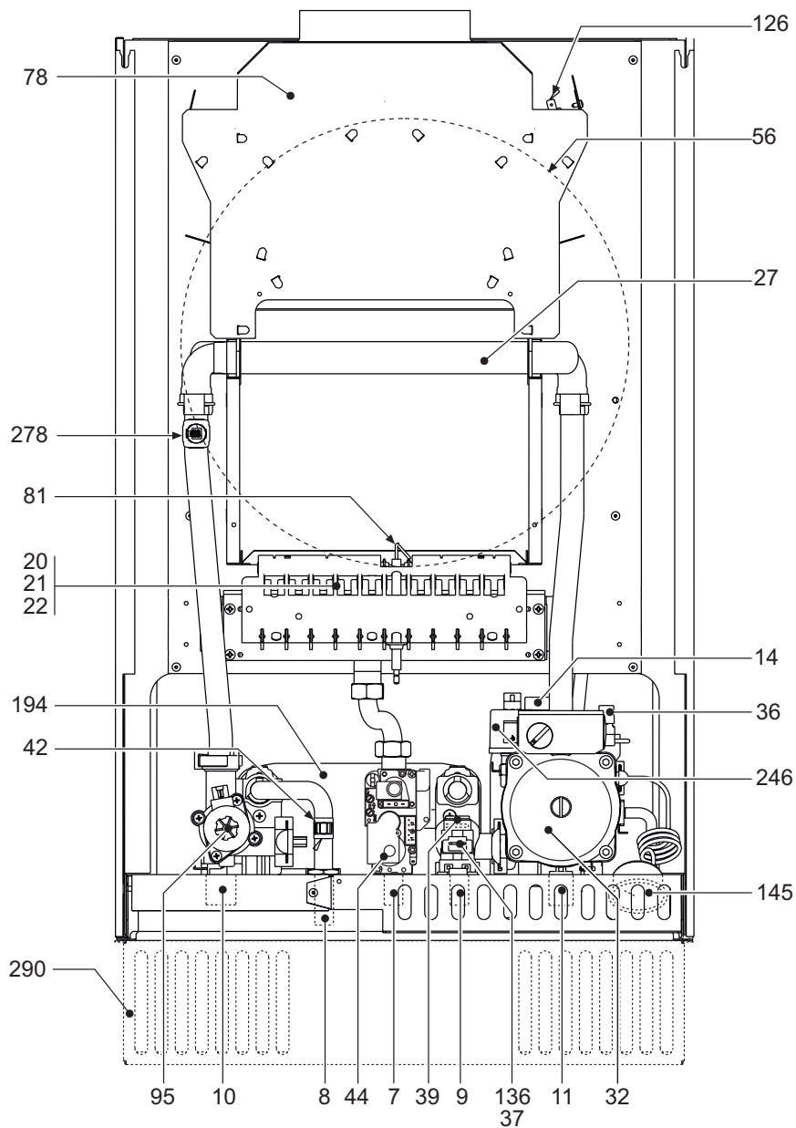
fig. 26 - Vista generale
