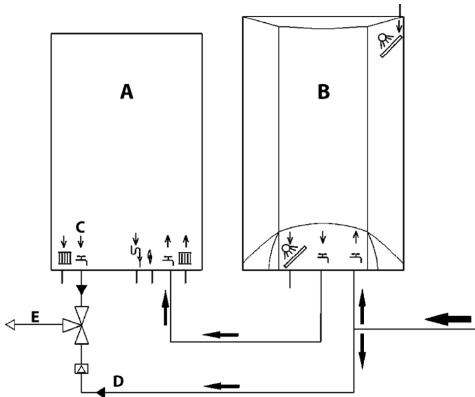
fig. 20 - Schema impianto solare
